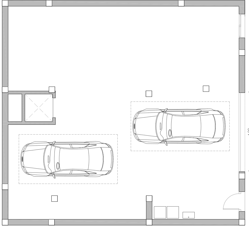
PLANTA SÓTANO
